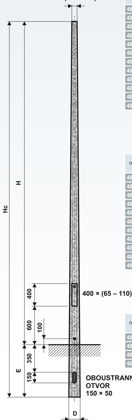
Průřez stožáru
